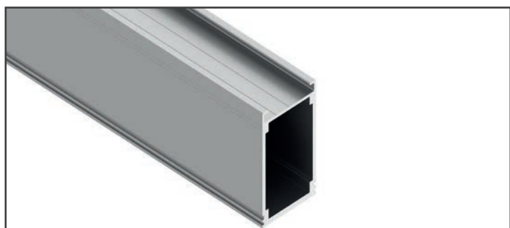
Alu HKP-Unterkonstruktion 60/100 mm
